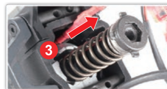
彈簧即可拿出，組裝步驟反之。
