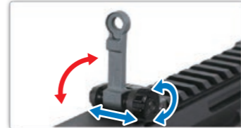
● Plegar y desplegar. ● Ajuste de viento (izquierda y derecha)
