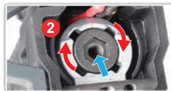
使用內六角(8mm)內壓頂桿之後轉動至開口處。
